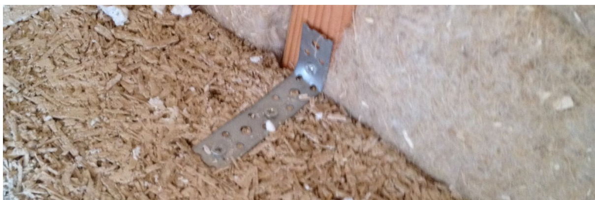
hoekijzer voor in houtskelet
